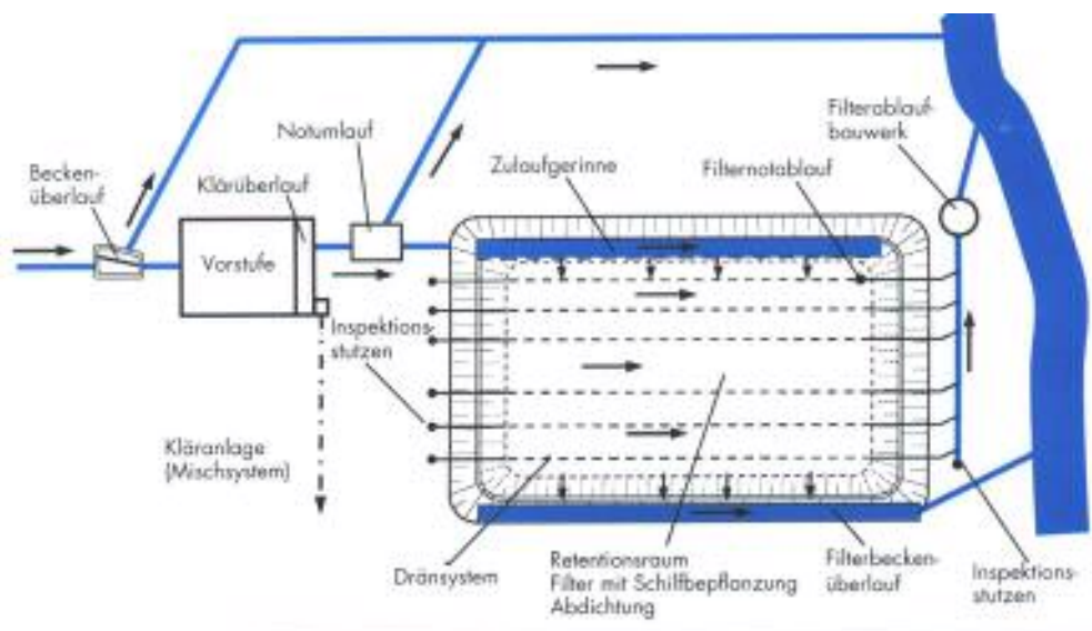
Prinzip eines Retentionsbodenfilters.
